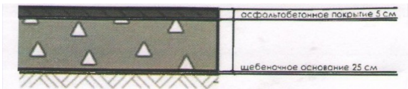
Устройство парковок
