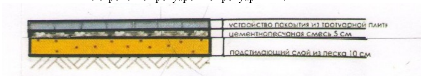
Устройство тротуаров из тротуарных плит
